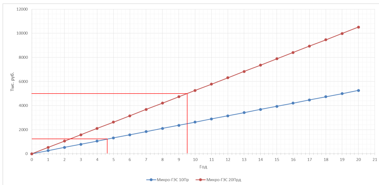
Рисунок 1 - Диаграмма окупаемости обоих гидрогенераторов
